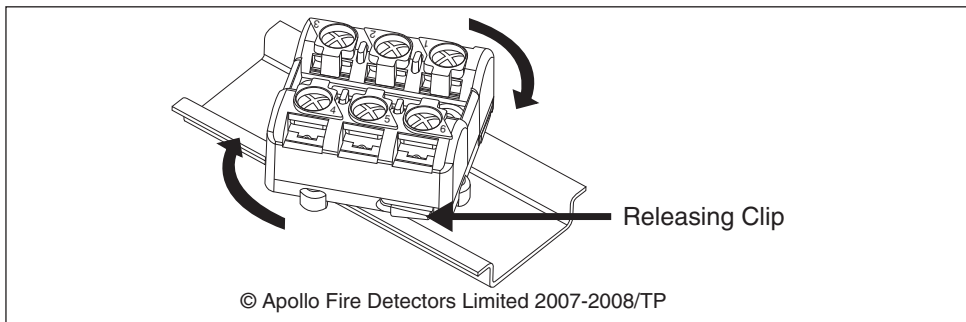
Fig 2 – Marine Mini Switch Monitor on a DIN Rail.
